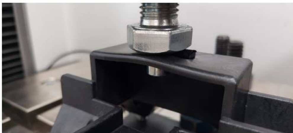
Dettaglio prova: dettaglio punto di rottura
